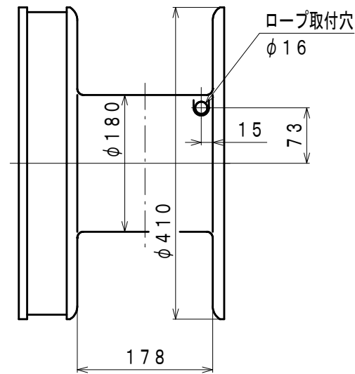
ドラム寸法
