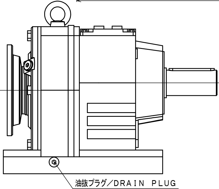
C矢視 / C-VIEW
