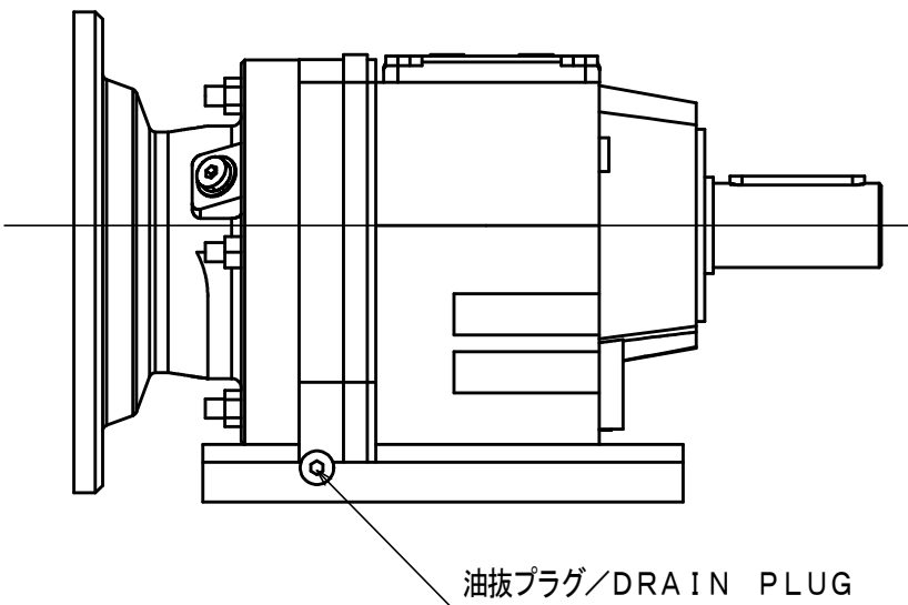
C矢視 / C-View
