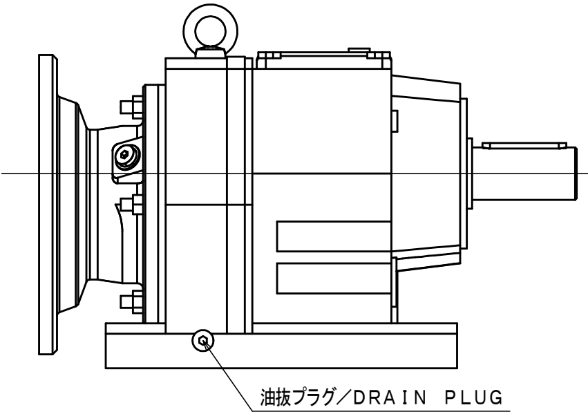
C矢視 / C-View
